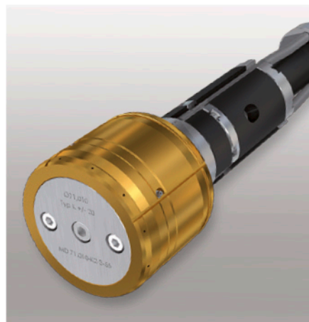
Gauging Mandrel
